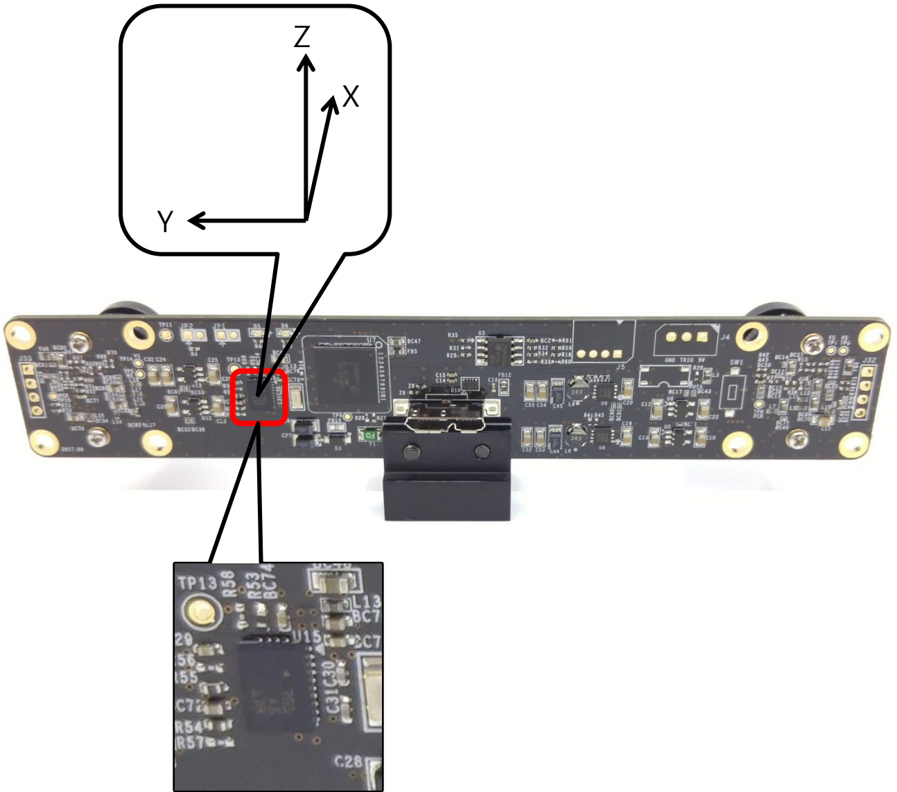
IMU Sensor
